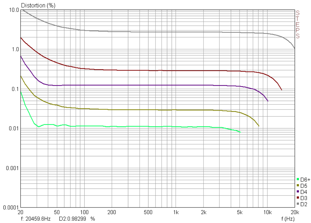
Vatse KT120 triode
