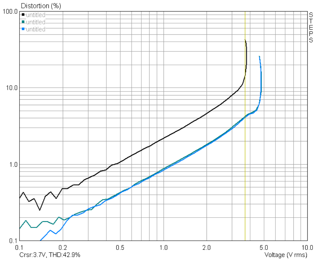
VATSE KT120 triode 30/1k/7k Hz
